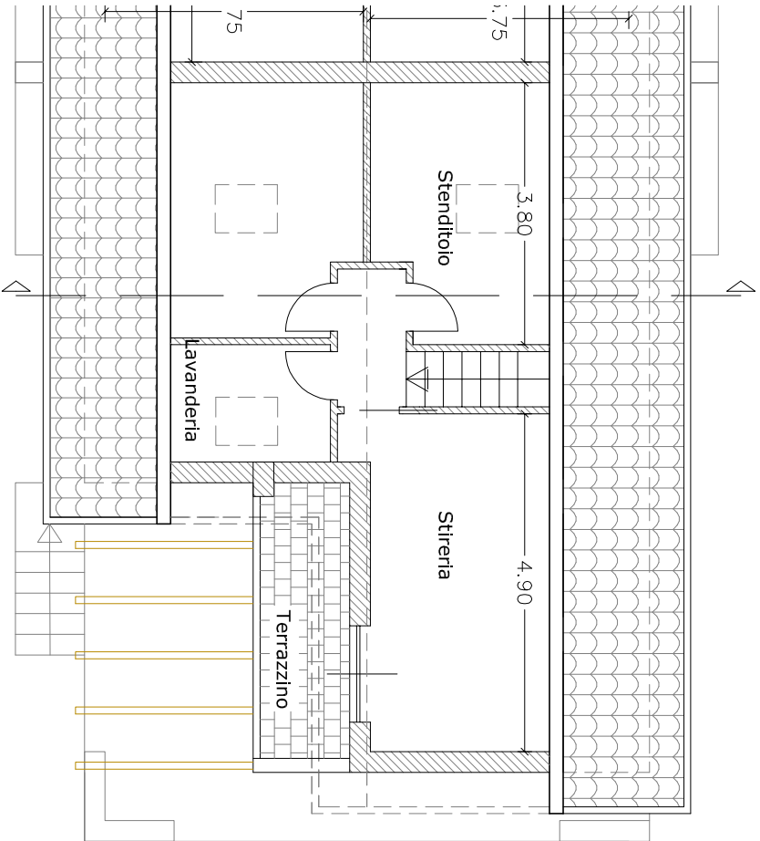
Pianta Piano Sottotetto Scala 1 : 100 Progetto
